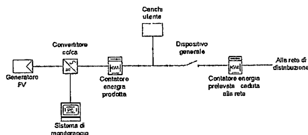
Schema a blocchi di un impianto collegato alla rete
