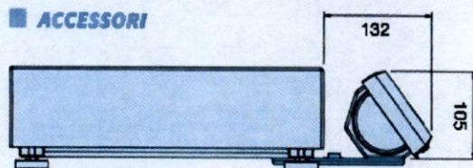
D 70 E per configurazione compatta su PMA
