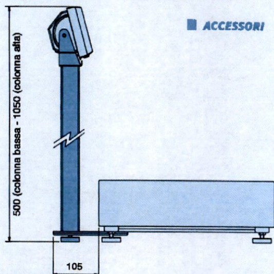
Colonna per applicazione su PMA
