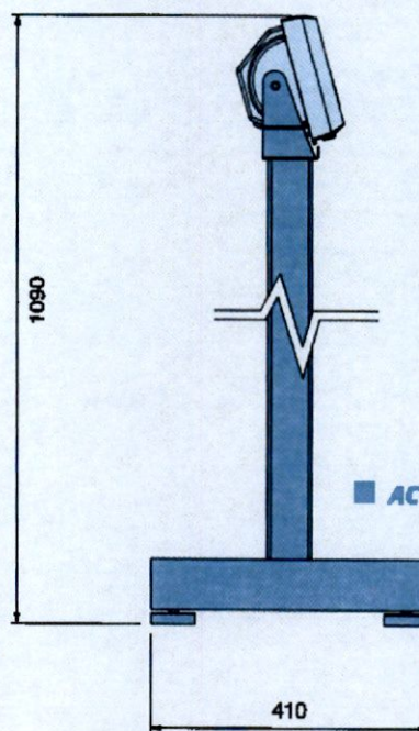
Colonna con piedistallo per collegamento a piattaforma di pesatura
