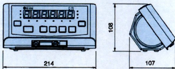
D 70 E versione da tavolo
