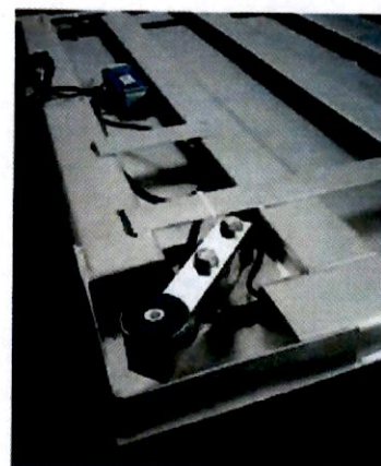
Alloggiamento della cella di carico (particolare)
