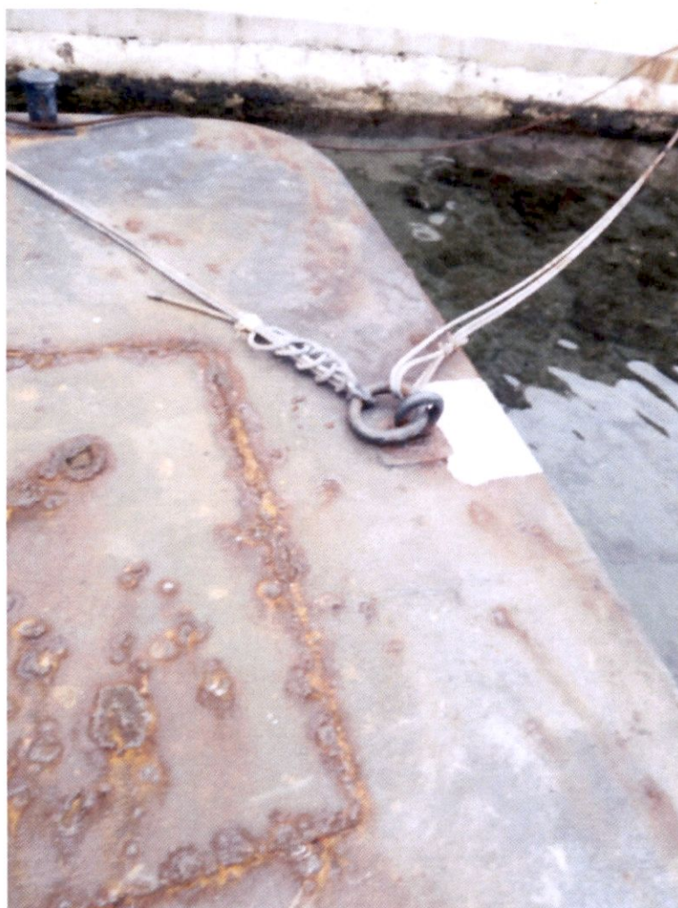
Ennesimo raddoppio di lamiera per la presenza di buchi in coperta
